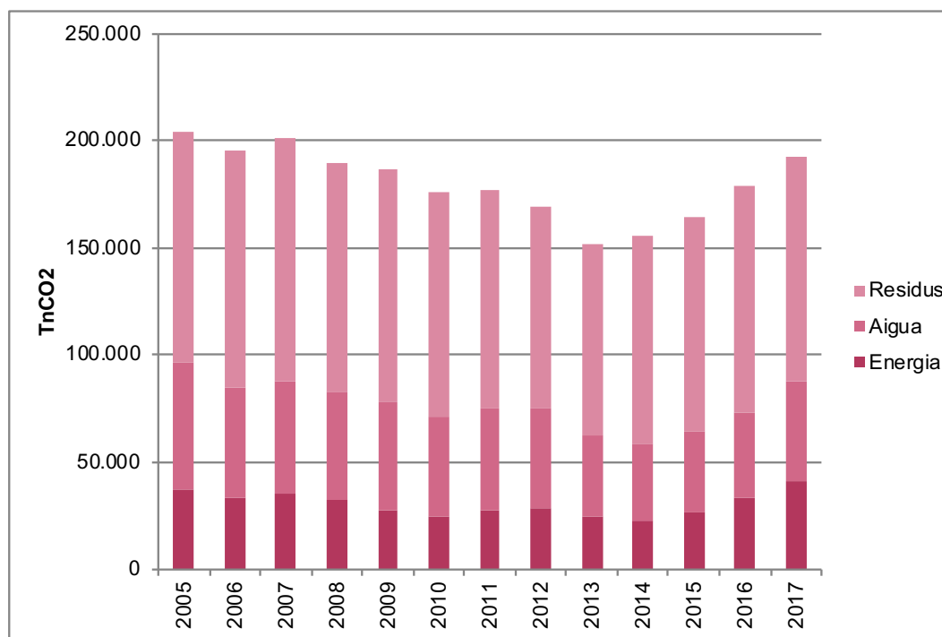
Gràfica evolució de les emissions de CO 2 a Viladecans. Sectors
